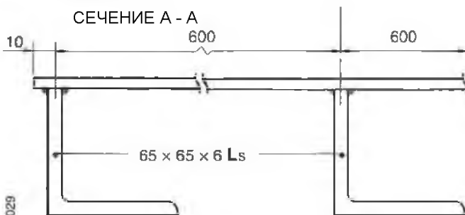
Фигура 1 - Сърцевина от структурна стомана за вертикална преграда от клас А и облицовка от клас В
