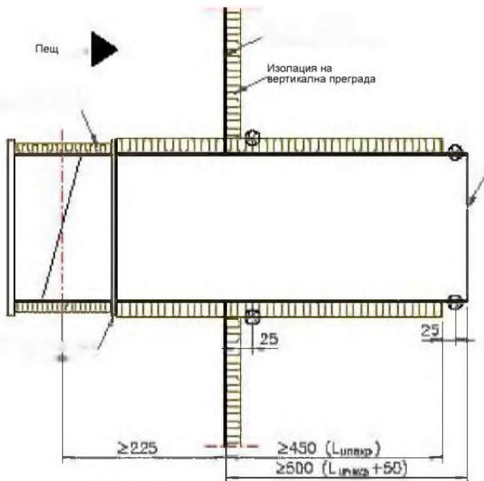
Образец от вертикална преграда
