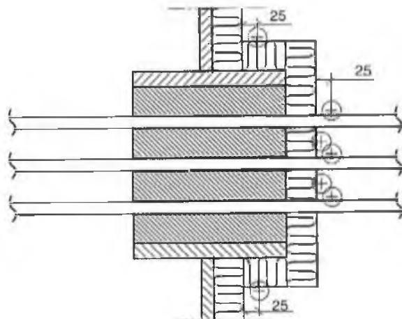
Фигура А2 - Проходи на кабели: положение на термодвойките с неизложена лицева страна (показано за вертикалната преграда)
