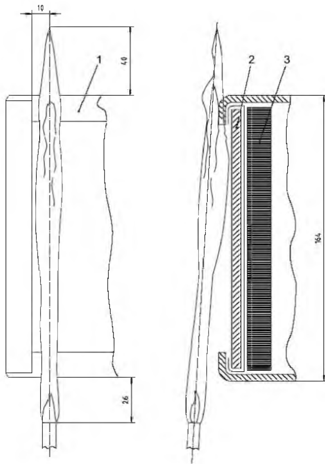
Фигура 6 - Разположение на пипотния пламък
