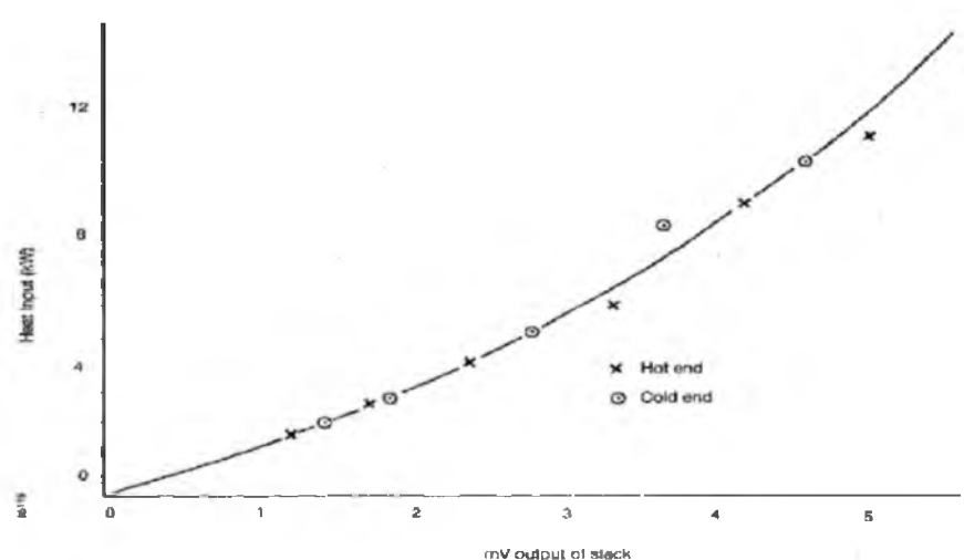
Фигура 9 - Пример за типично калибриране със стек
