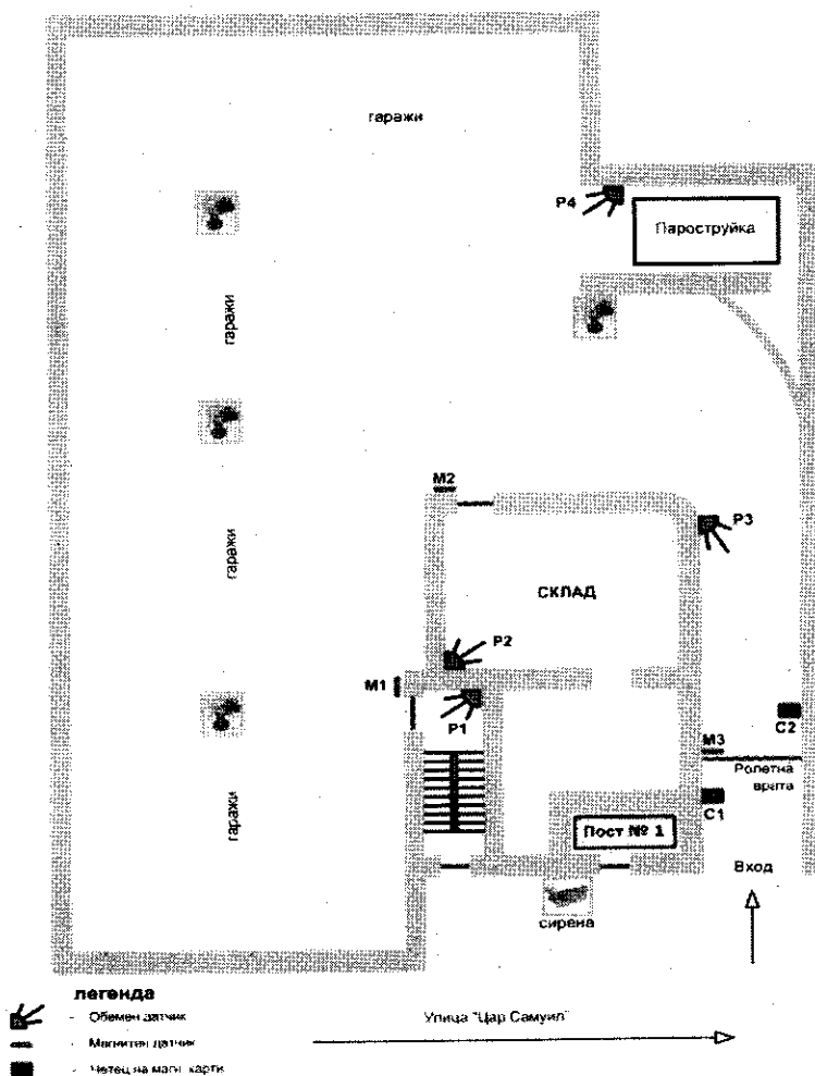
СХЕМА на разположението и техническото оборудване на Обект “Подземен гараж”
